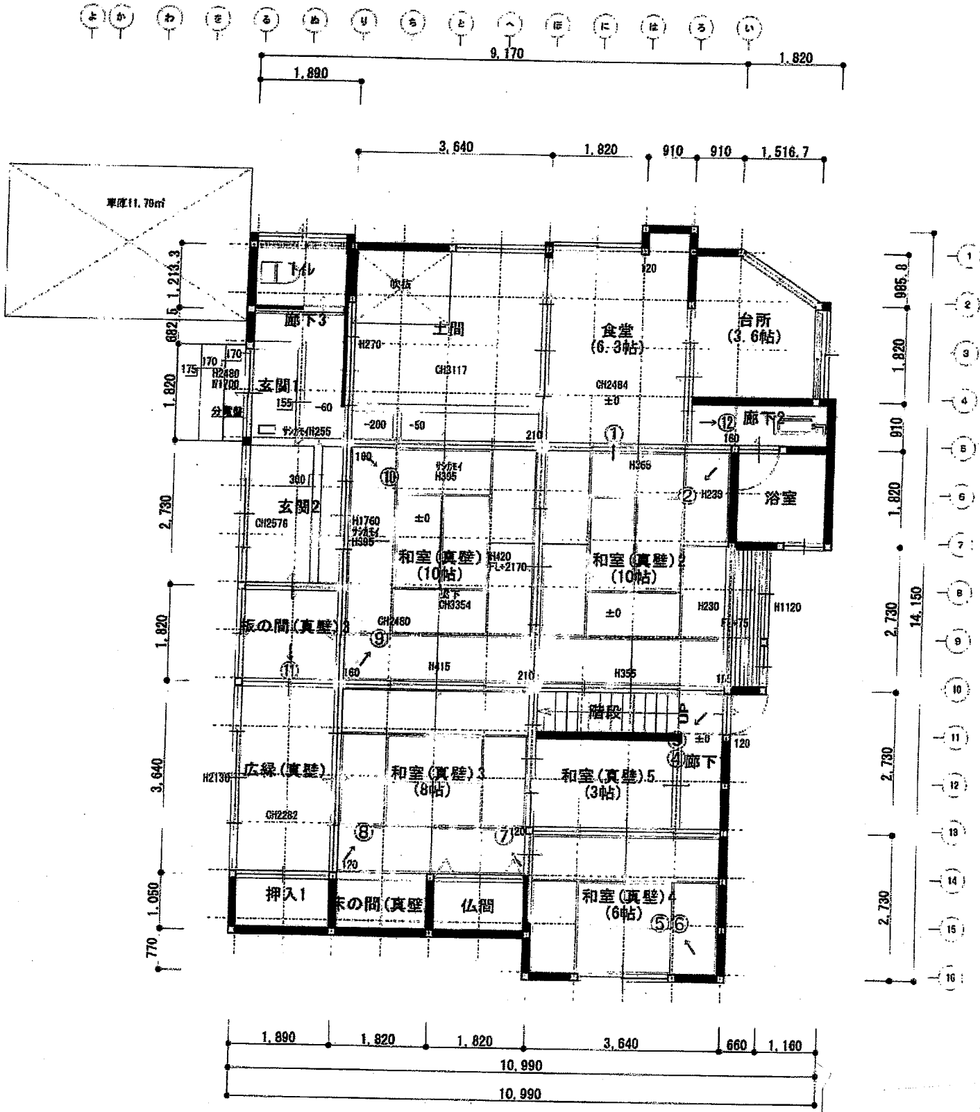
1F 既存平面図
