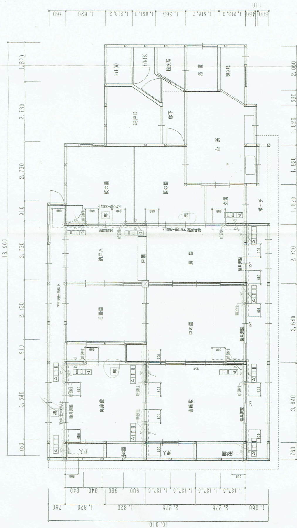
改修1階平面図 S=1/70
