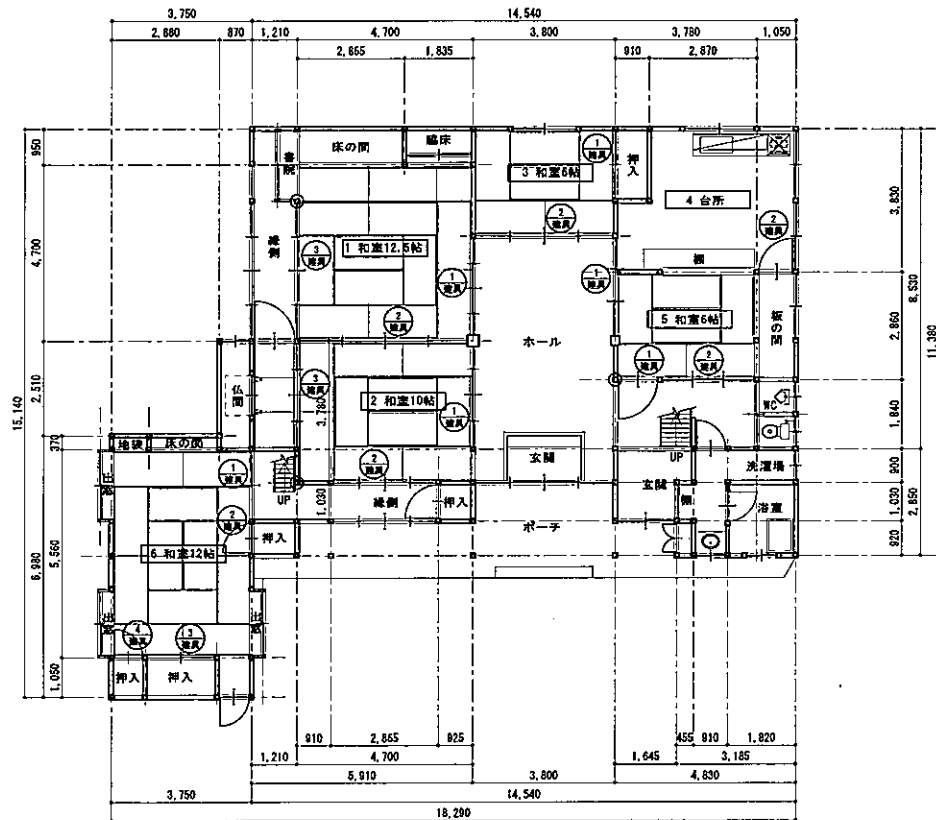
1階平面図 (5=1/100)
